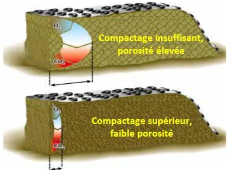
Figure 1 : Impact du compactage sur l'infiltration d'air (Mahanna, 2018)
